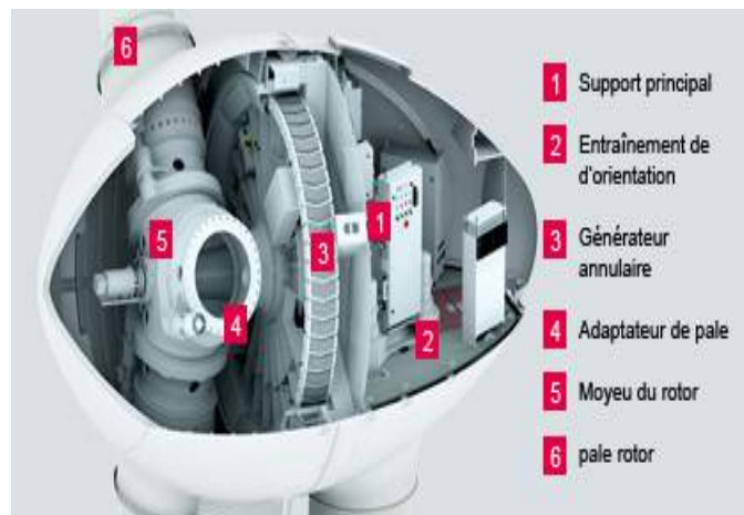
Figure 7 : coupe transversale de la nacelle E53
