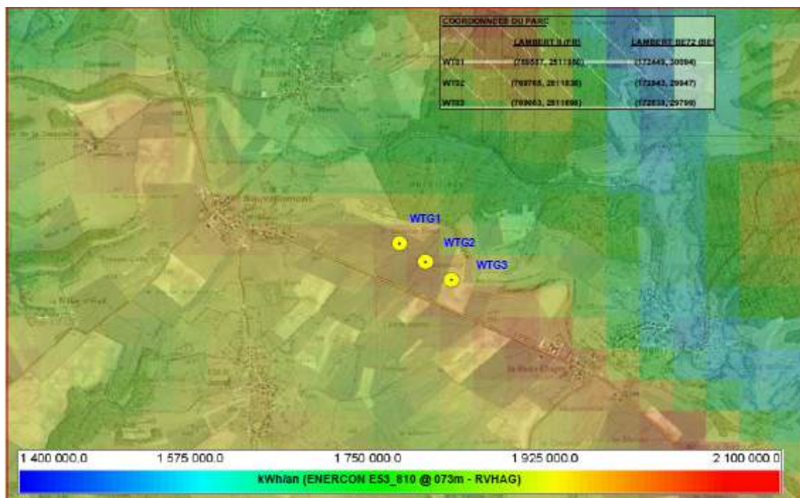
Figure 2 : Cartographie de l'estimation de production du parc (Atm-Pro 2013)
