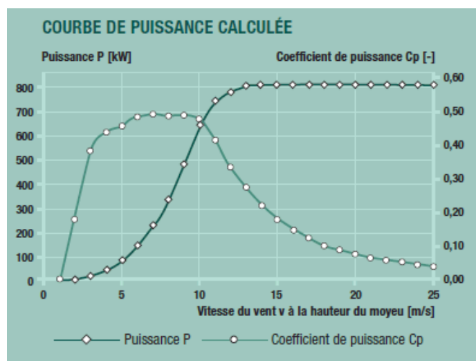
Figure 8 : courbe de puissance E53
